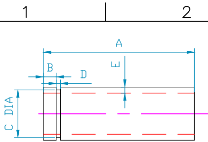
RING GROOVE DIMENSIONS
